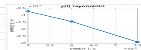
Сурет 7 – MatLab
